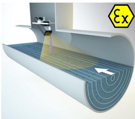
Abb. 2: Kombinierte Sensoreinheit
