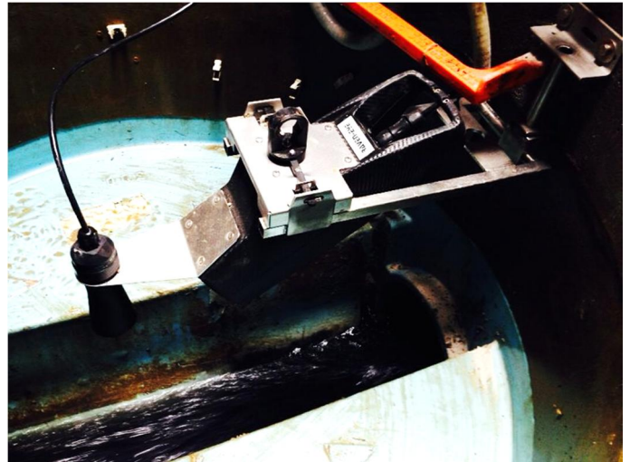
Abb. 1: Berührungslose Sensorik im Kanal
